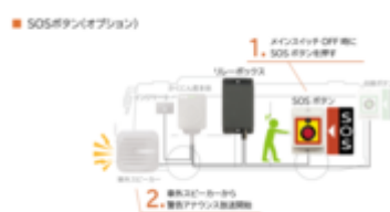
システム機器構成(SOSボタン)
